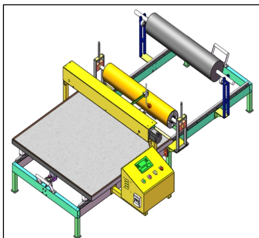
SBS 改性沥青卷材恒定热熔试验机
